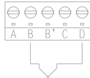
热电偶
