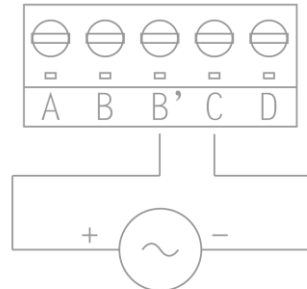
电流0~20mA
