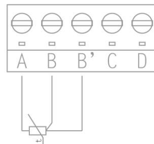
Pt100三线制
