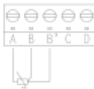
Pt100三线制
