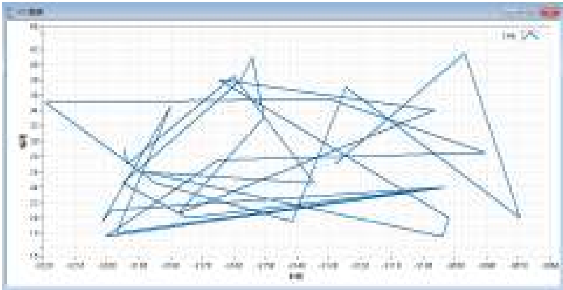
XY图表
